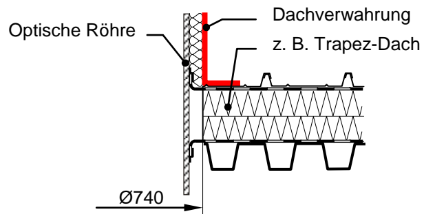
Detail: Dachöffnung
