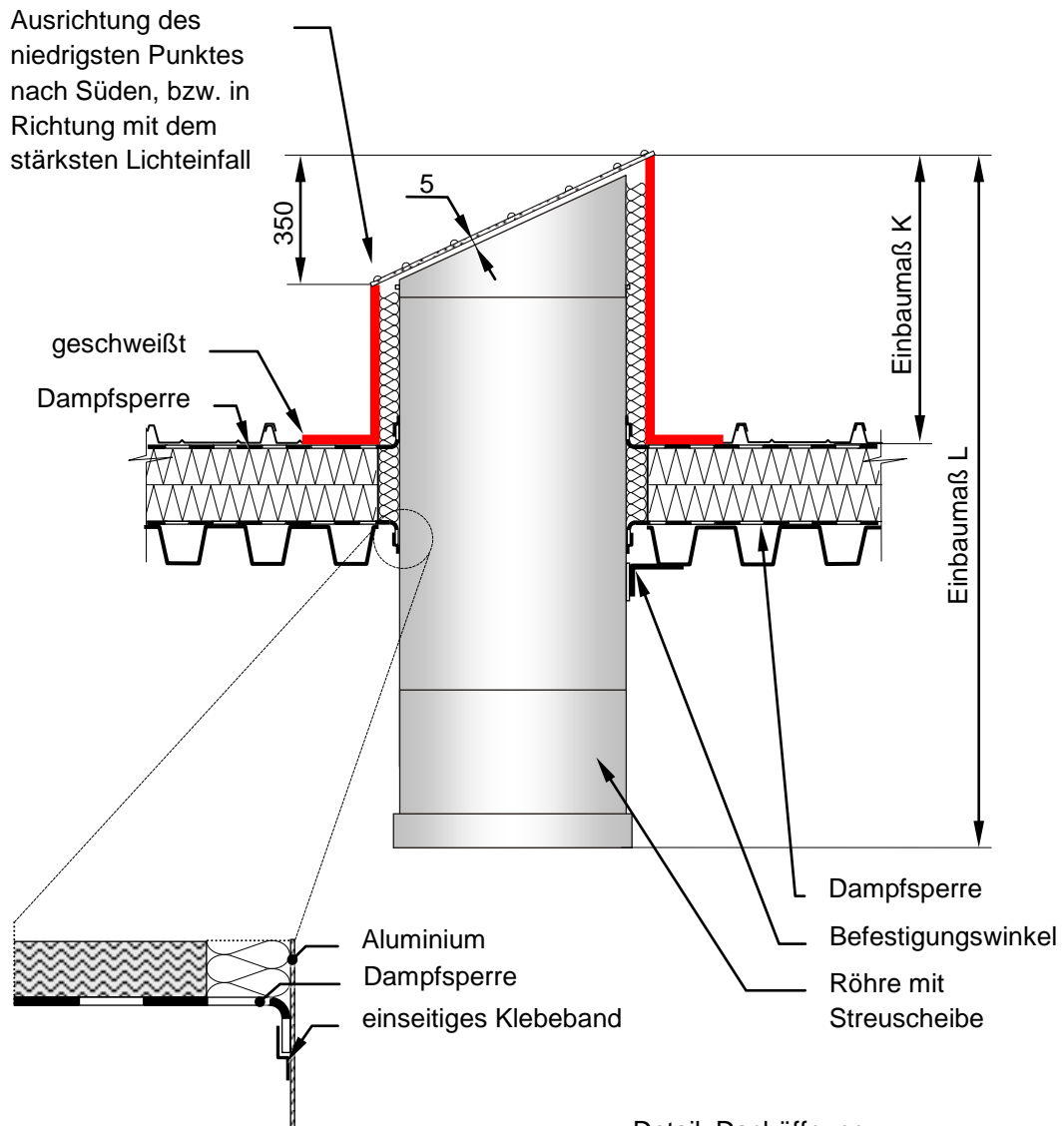
Detail: Dachöffnung
